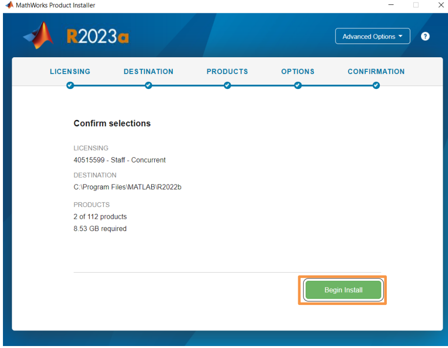
Şekil 13: Doğrulama Ekranı
