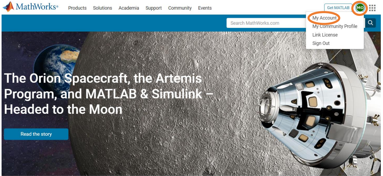
Şekil 1: Hesaba giriş
