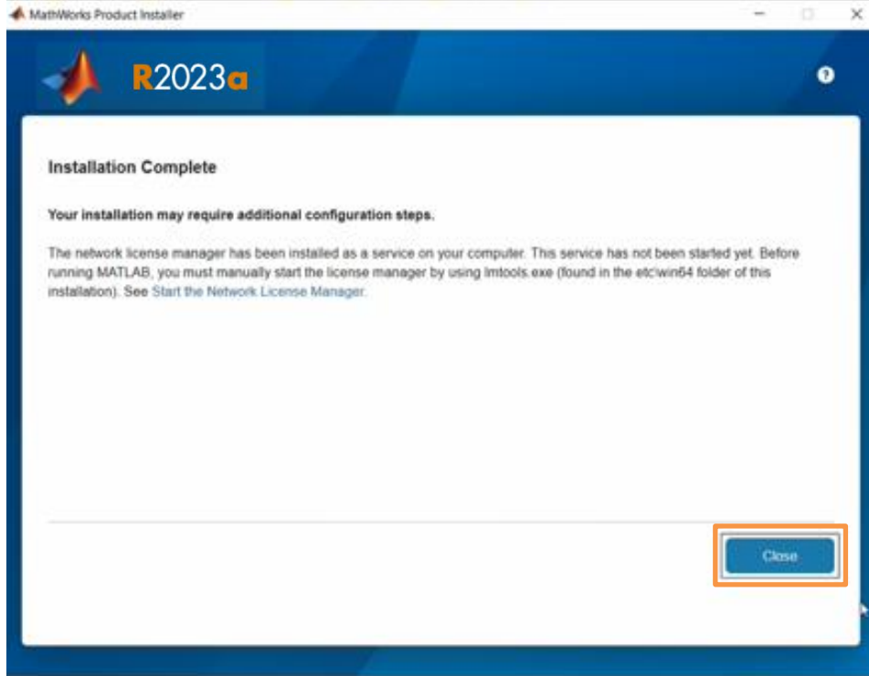
Şekil 14: Yükleme tamamlandı
