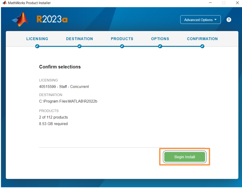
Şekil 24: Doğrulama Ekranı
