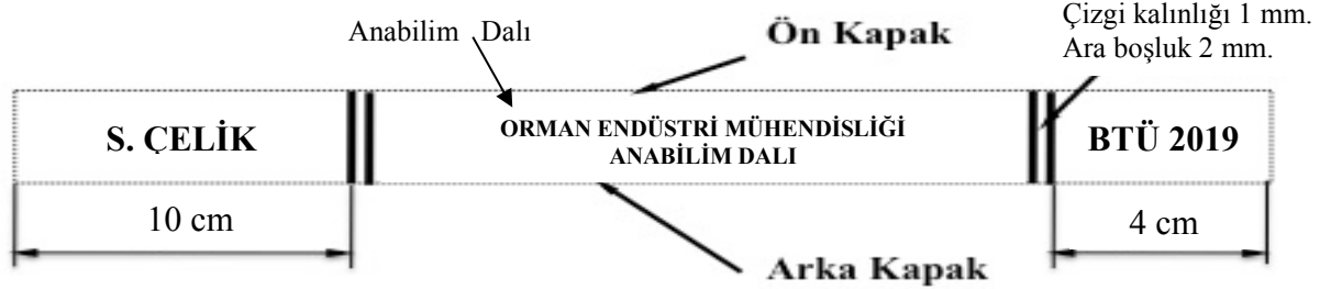
Şekil 2.2: Bez cilt dış kapak sırtının düzeni ve boyutları.
